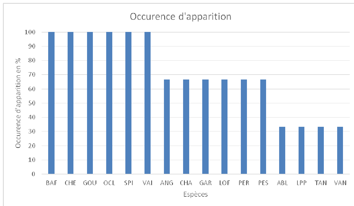
Figure 11. Fréquence d'apparition des espèces de poisson sur la station Lavaux1
